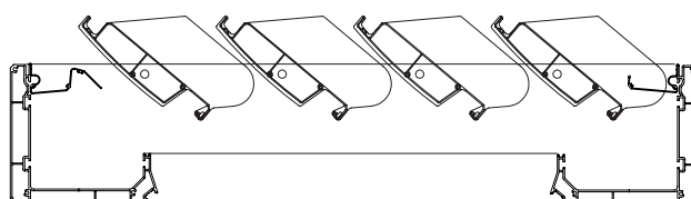
Rotation lames à 140°
