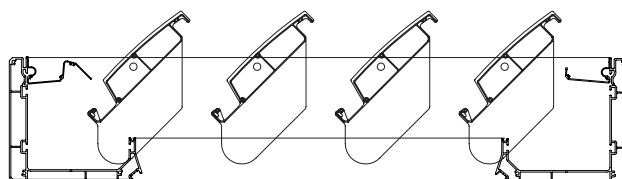
Rotation lames à 45°
