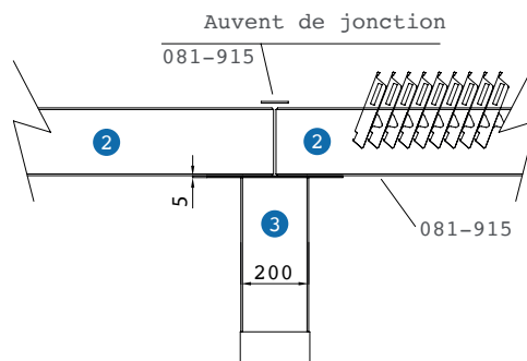
Vue latérale.
