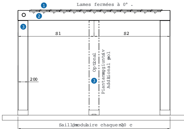
Vue latérale
