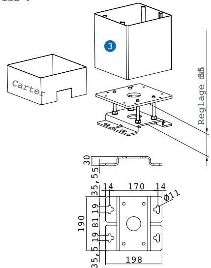
Pied .
