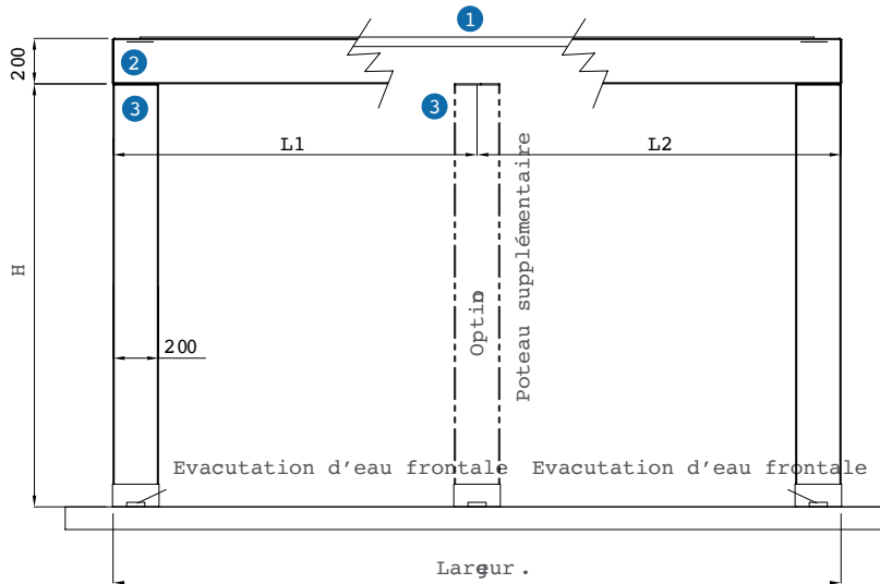
Vue frontale
