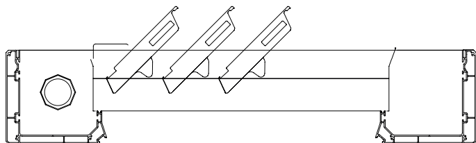
ouverture progressive 45° .
